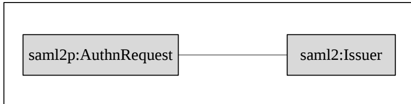
Рисунок 7 – Структура AuthnRequest
