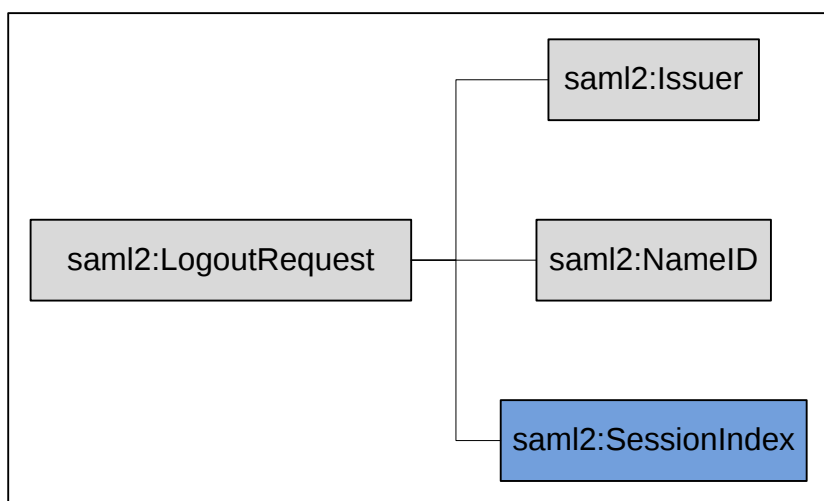
Рисунок 11 – Структура LogoutRequest
