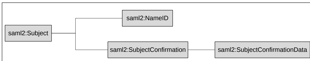
Рисунок 9 – Структура saml2:Subject
