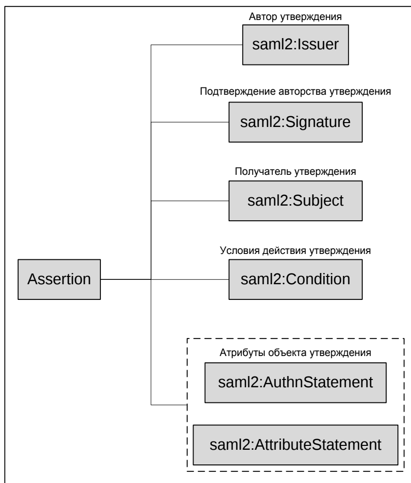
Рисунок 8 – Структура AuthnResponse
